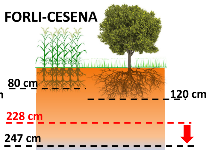
LIVELLI DI FALDA CONFRONTO ANNO
