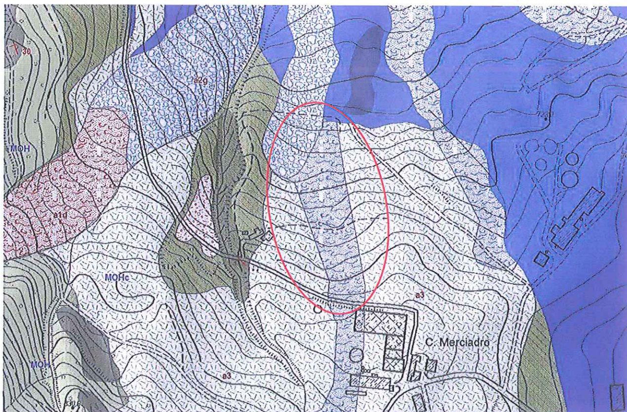
Fig. 5.1-1- Estratto Carta Geologica Regione Emilia – Romagna scala 1:5.000
