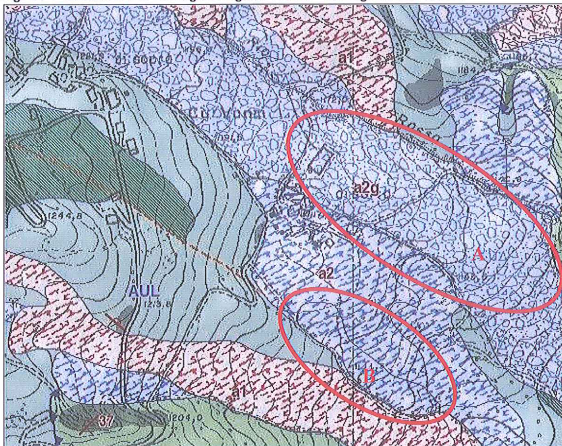
Fig. 5.1-1- Estratto Carta Geologica Regione Emilia – Romagna scala 1:5.000
