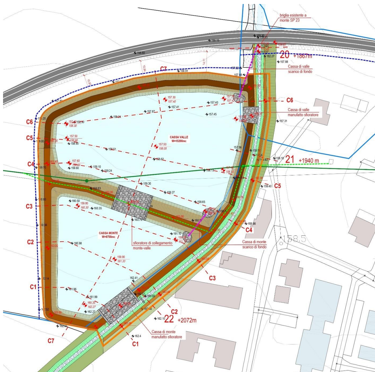
FIGURA 2-2 – SCHEMA PLANIMETRICO DEGLI INTERVENTI DI PROGETTO
