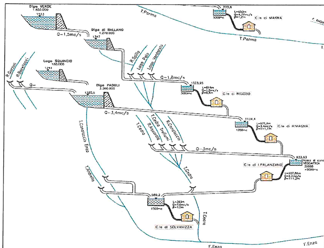
Figura 2: Schemi ENEL presenti sul bacino dell'Enza (immagine tratta da pubblicazioni ENEL)
